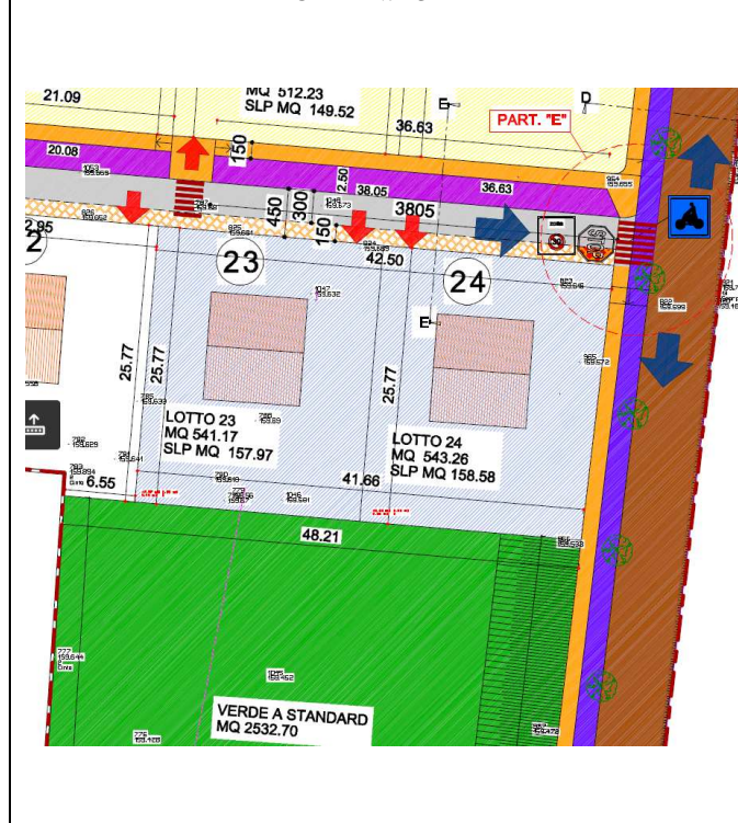
ESTRATTO DEL PIANO DI LOTTIZZAZIONE ART "A" LOTTI N. 23 E 24
