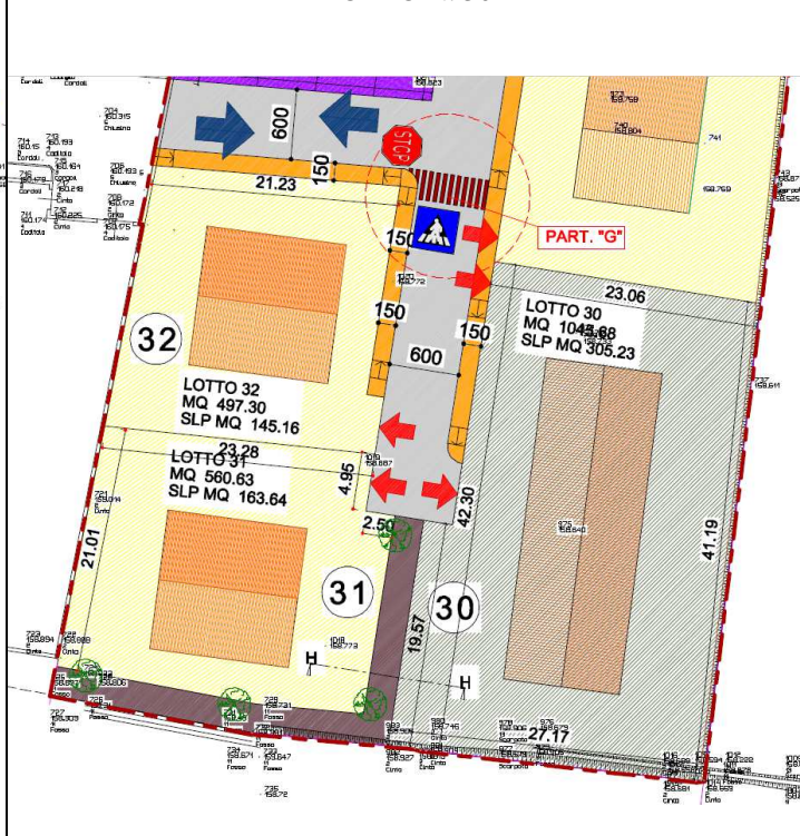
ESTRATTO DEL PIANO DI LOTTIZZAZIONE ART "A" LOTTO N. 30
